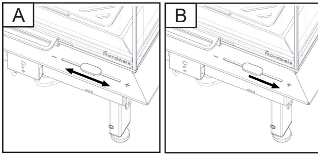
Zündluftregler
